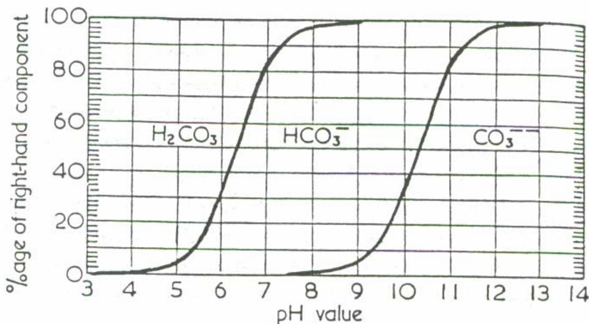
شکل ۱۴- تعادل کربنات ، بی کربنات و اسید کربنیک با PH
